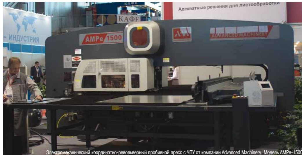
Электромеханический координатно-револьверный пробивной пресс с ЧПУ от компании Advanced Machinery. Модель AMPe-1500
